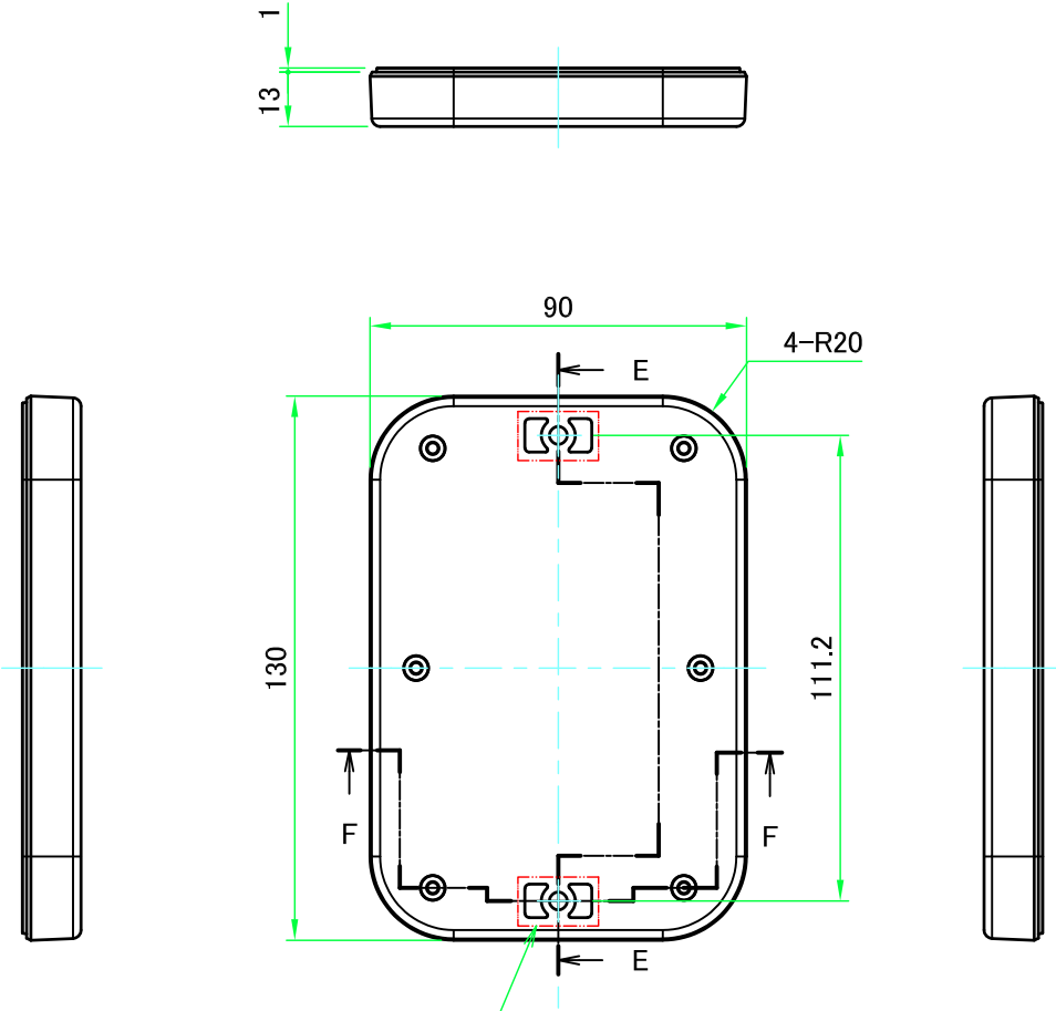
2-ポールマウントブラケット(WPMB-M4)用取付ガイド 2-Mounting position for Pole Mounting Bracket (WPMB-M4)
